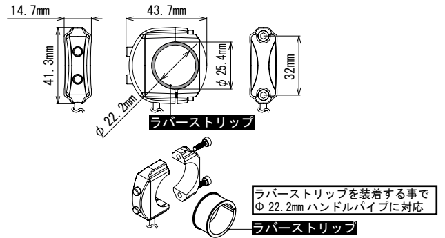
メーター外部スイッチ寸法図
