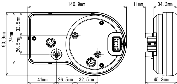
メーター本体寸法図
